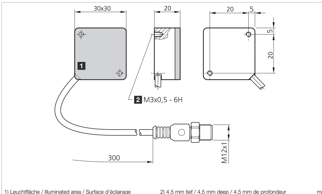
1) Leuchtfläche / Illuminated area / Surface d'éclairage 2) 4.5 mm tief / 4.5 mm deep / 4.5 mm de profondeur mm
