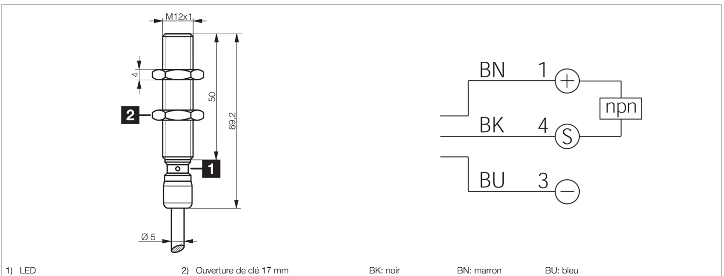
1) LED 2) Ouverture de clé 17 mm BK: noir BN: marron BU: bleu
