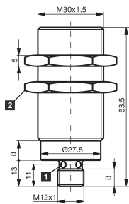
1) LED 4 x 90° (jaune) 2) Ouverture de clé 36 mm BN: marron BU: bleu WH: blanc
