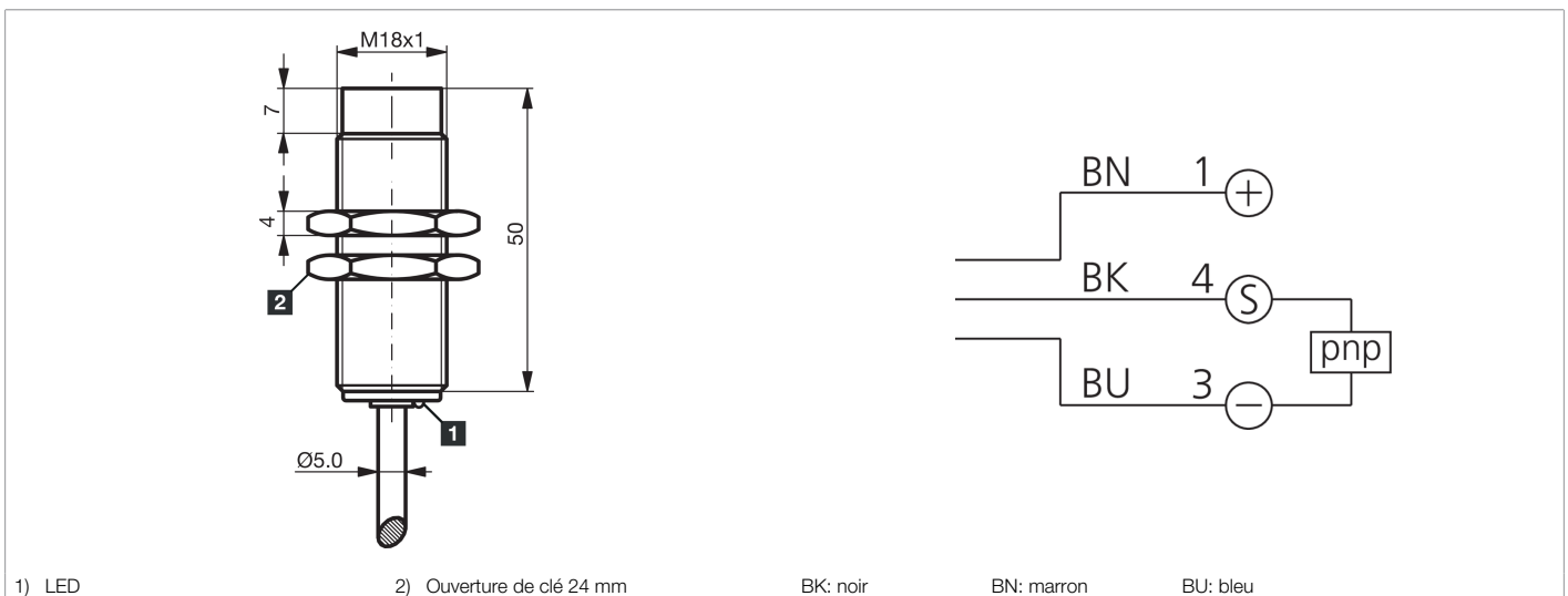
1) LED 2) Ouverture de clé 24 mm BK: noir BN: marron BU: bleu
