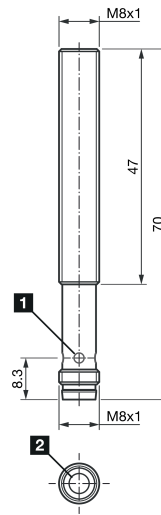
1) LED 4 x 90° (gelb) / LED 4 x 90° (yellow) / LED 4 x 90° (jaune) 2) Schallaustritt Ultraschallwandler / Sound outlet ultrasonic transducer / Sortie sonore transducteur à ultrasons mm
