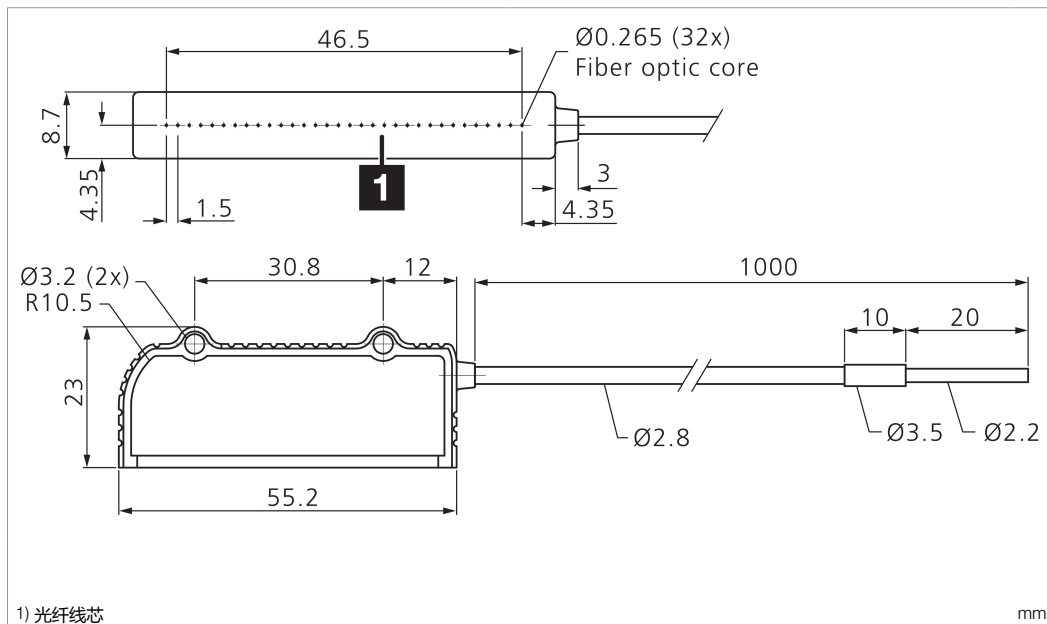
1) 光纤线芯
