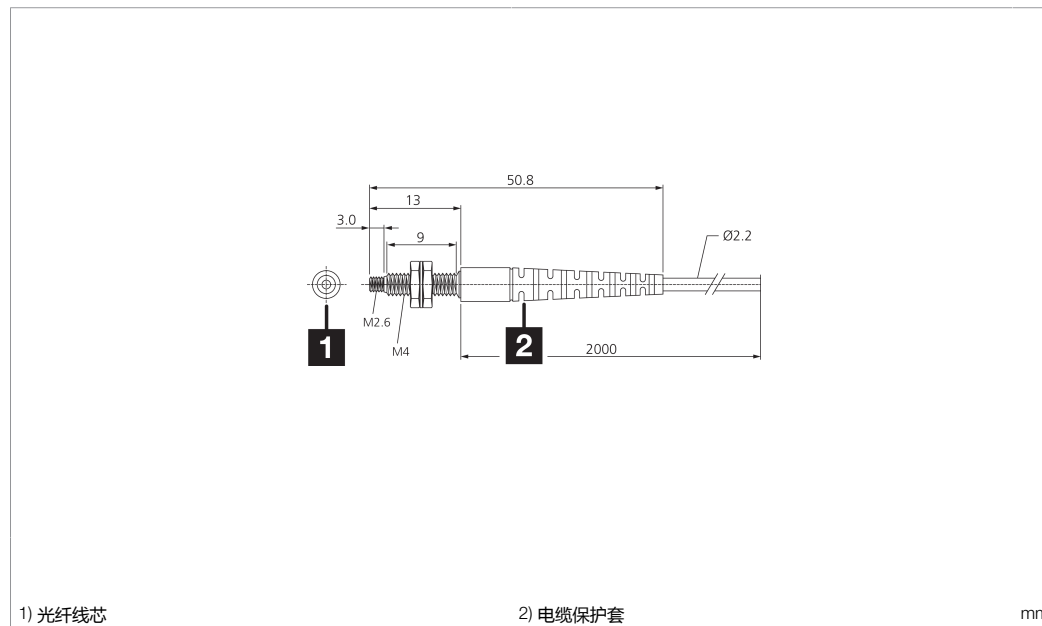
1) 光纤线芯
