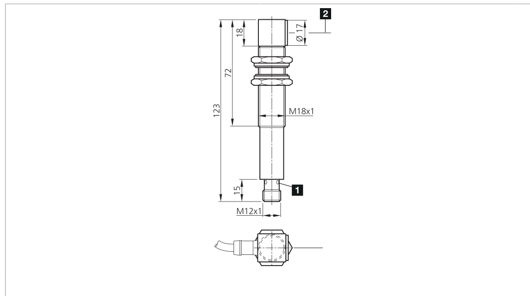
1) LED 4 x 90° (gelb) / LED 4 x 90° (yellow) / LED 4 x 90° (jaune) 2) Schallaustritt Ultraschallwandler / Sound outlet ultrasonic transducer / Sortie sonore transducteur à ultrasons mm
