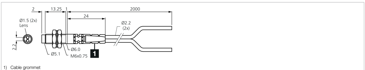
1) Cable grommet
