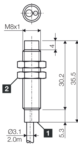
1) LED 2) Schlüsselweite 13 mm BK: schwarz BN: braun BU: blau
