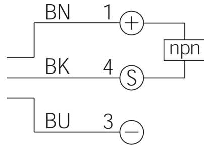
1) LED 2) Schlüsselweite 13 mm BK: schwarz BN: braun BU: blau
