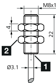
1) LED 2) Schlüsselweite 13 mm BK: schwarz BN: braun BU: blau
