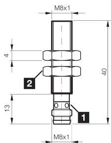
1) LED 4 x 90° (gelb) 2) Schlüsselweite 13 mm BK: schwarz BN: braun BU: blau
